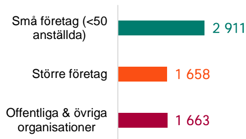
Antal jobb per sektor i Malung-Sälens kommun 2022
